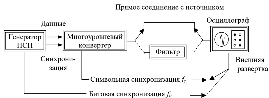
Рисунок 1 – Построение глаз-диаграммы
