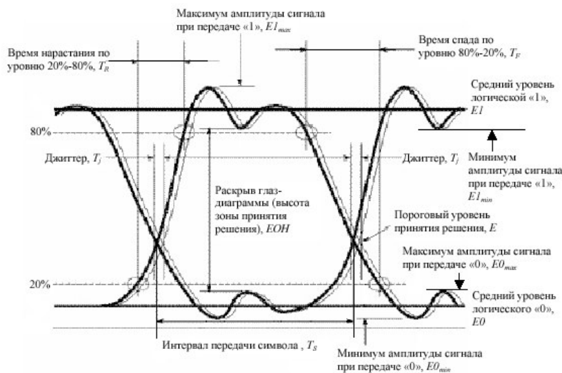
Рисунок 2 – Идентификация глаз-диаграммы
