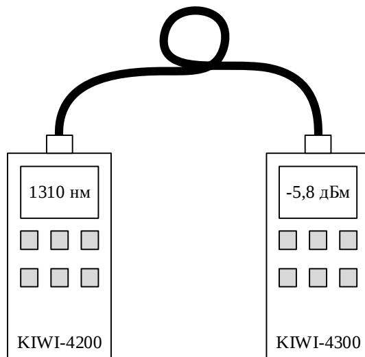
Рисунок 1 – Схема соединения источника и приемника оптической мощности
