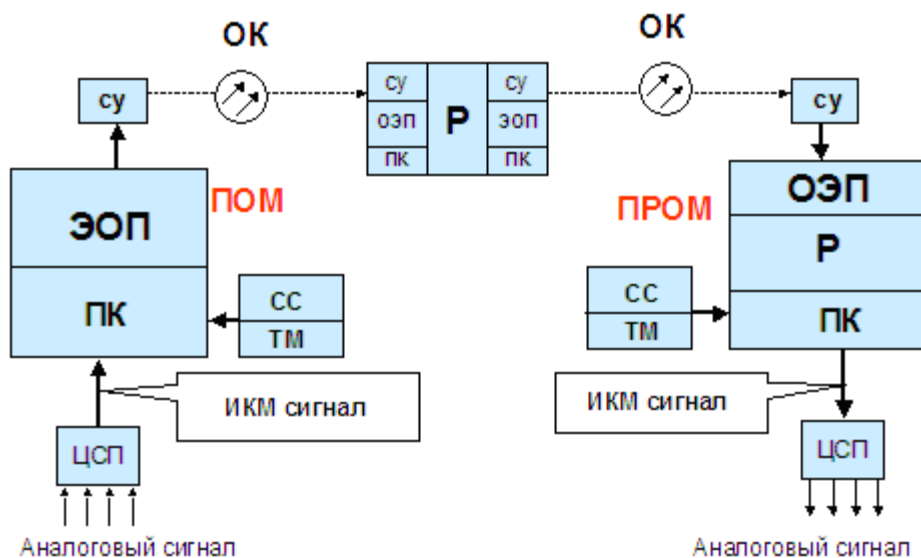
Обобщенная структурная схема ВОСП
