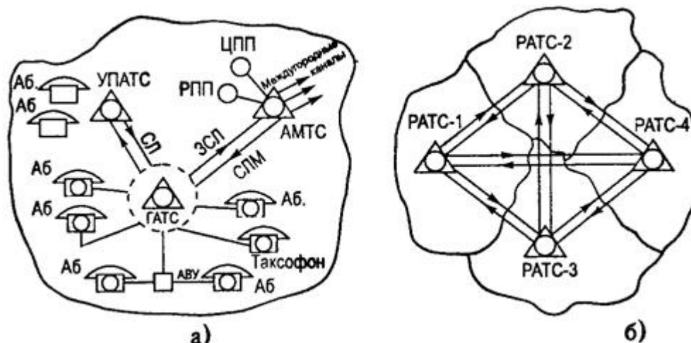
Структурная схема нерайонированной (а) и районированной (б) ГТС без узлов
