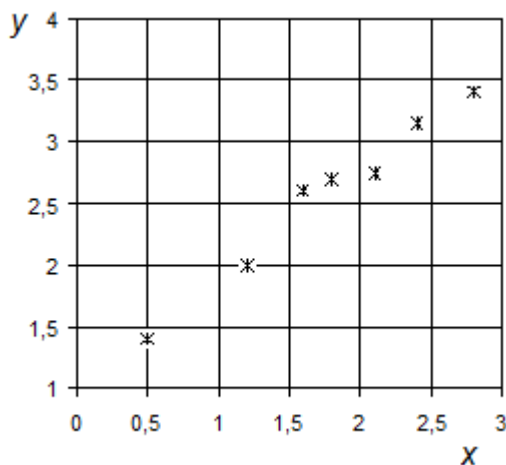
График заданной совокупности значений X и Y
