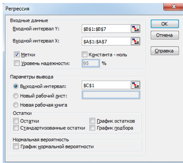
Рисунок 3.2 – Диалоговое окно ввода данных и параметров вывода
