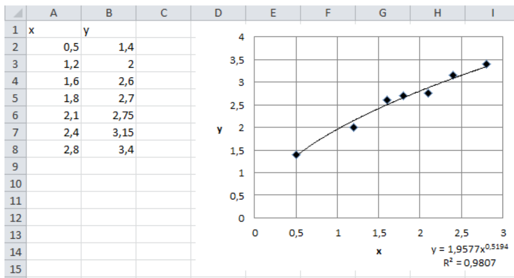
Рис. 3 - График заданной совокупности значений X и Y и линии тренда
