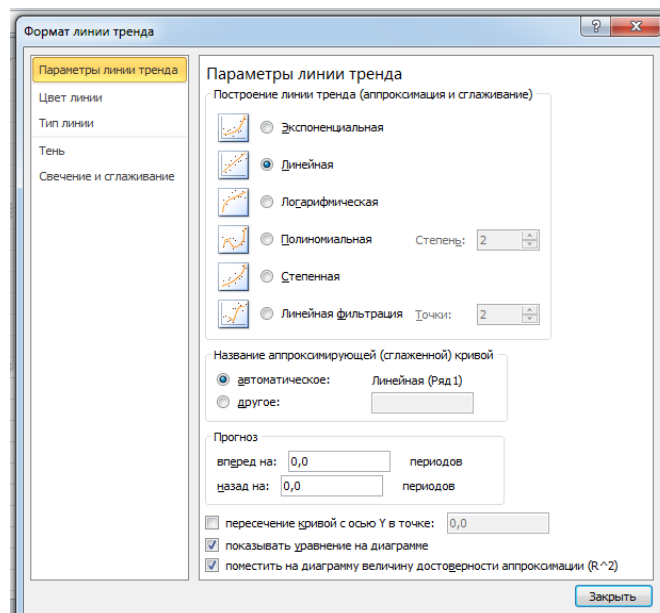
Рис. 2 - Диалоговое окно параметров вывода данных
