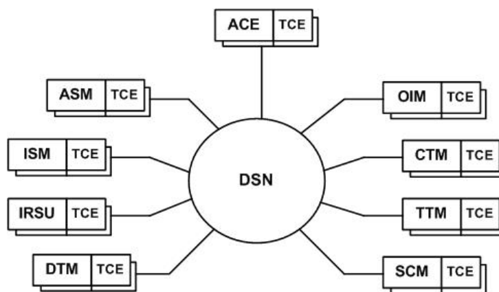
Рисунок 1.1 – Структурная схема ЦСРС S-12
