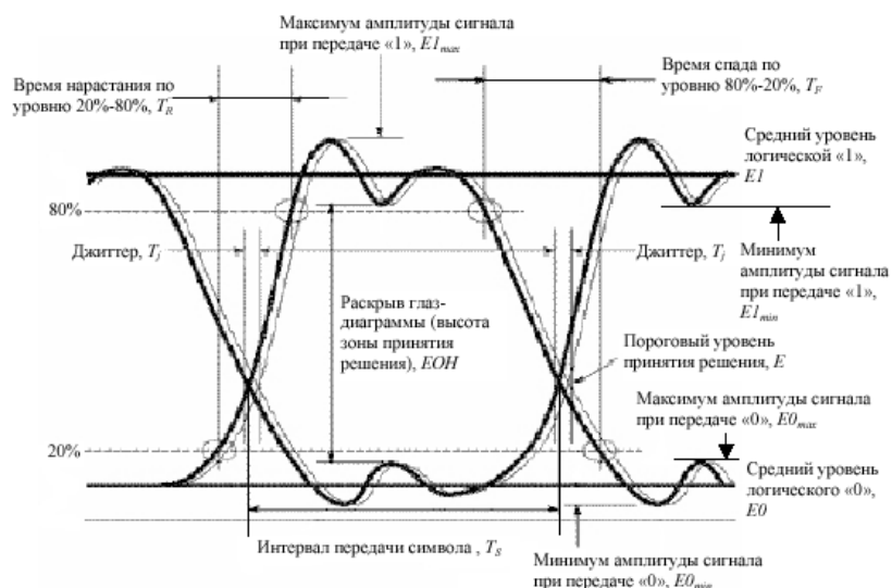
Рисунок 2 – Идентификация глаз-диаграммы
