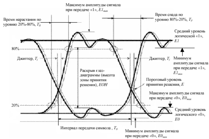
Рисунок 2 – Идентификация глаз-диаграммы
