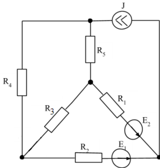
Рисунок 5 – Схема для расчета методом уравнений Кирхгофа
