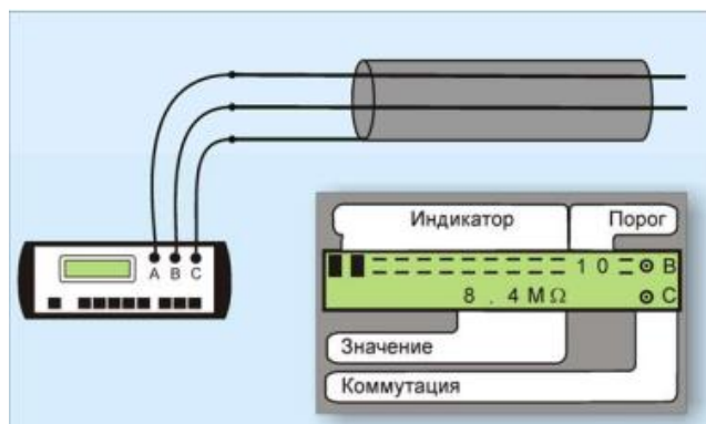
Рисунок 7 - Схема измерения сопротивления изоляции
