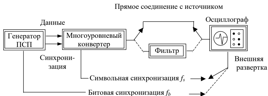
Рисунок 1 – Построение глаз-диаграммы
